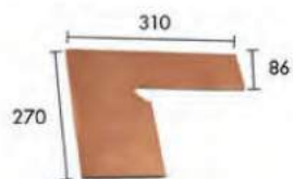
ZANQUÍN VIERTEAGUAS
