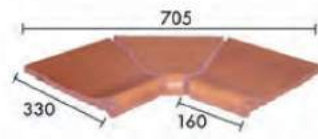
(*) CARTABÓN BORDE PISCINA INTERIOR
