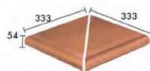
CARTABÓN PELDAÑO FIORENTINO
