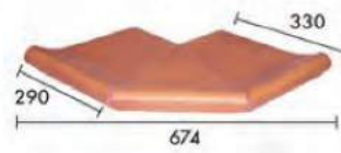
(*) CARTABÓN BORDE PISCINA EXTERIOR
