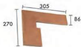
ZANQUÍN RECTO
