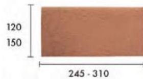
LOSETA CORTE
